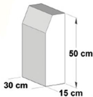
E 5030 وزن ۵۴ کیلوگرم
