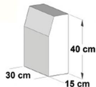
E 4030 وزن ۴۲ کیلوگرم
