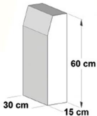
E 6030 وزن ۶۴ کیلوگرم
