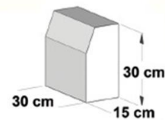
E 3030 وزن ۳۳ کیلوگرم
